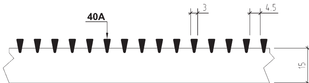
SEZIONE B-B
