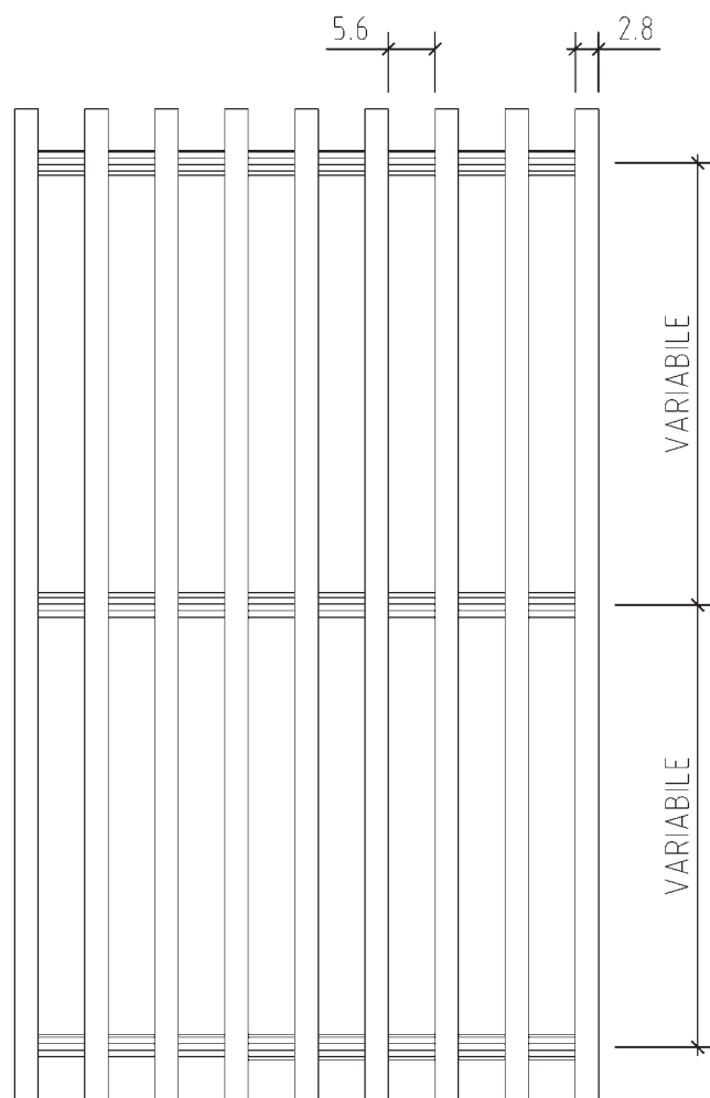
ESEMPIO 34S/D
