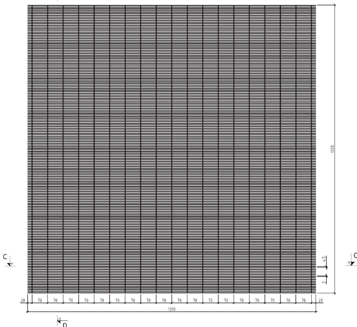
PROSPETTO PIANEROTTOLO
