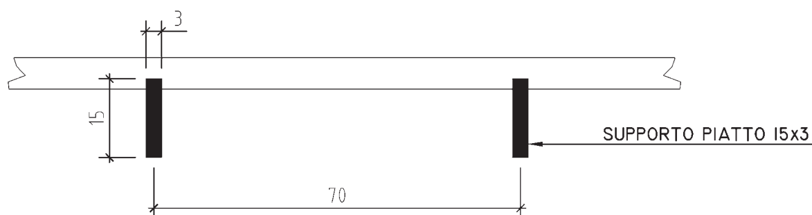
SEZIONE A-A
