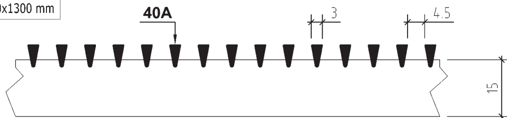
SEZIONE D-D
