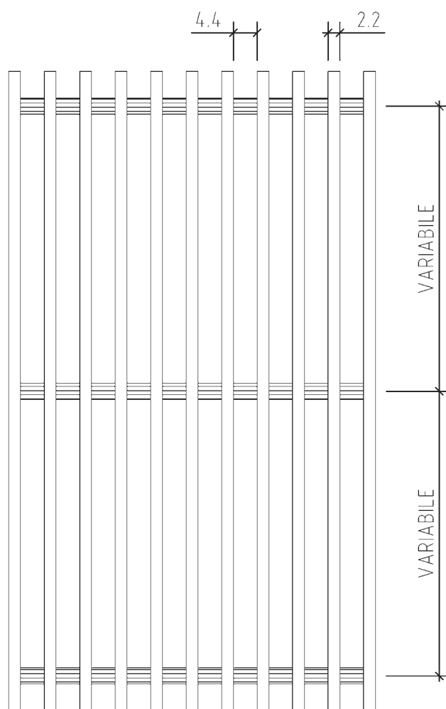
ESEMPIO 28S/D
