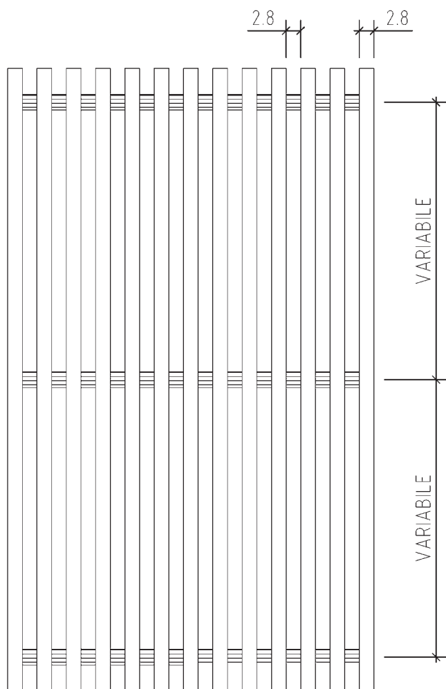
ESEMPIO 34S/A
