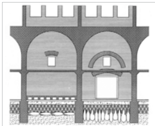
Esempio di fondazione ventilata al tempo dei romani.
