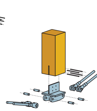
Tensione inferiore
