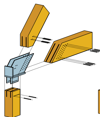
Giunto d'appoggio
