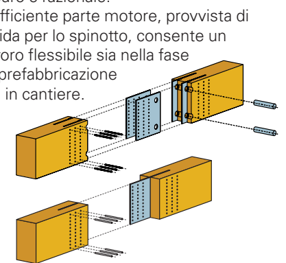
Giunzione ad incastro / Ristrutturazione
