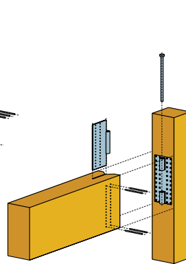
Giunzione Pilastro/trave
